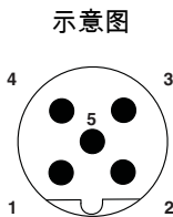
M12针式连接器引脚分配, 5芯, B编码, 插头侧
