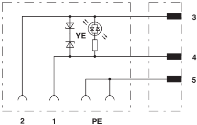
电路图
