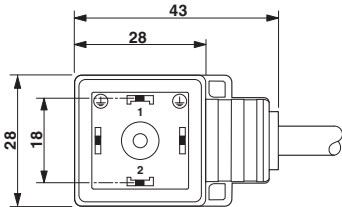
尺寸图
