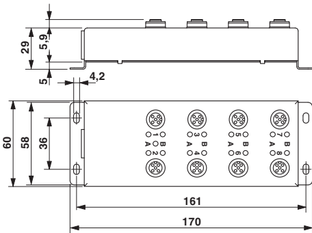
尺寸图
