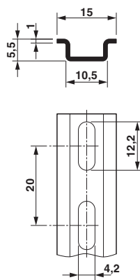
尺寸图
