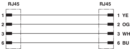
电路图
