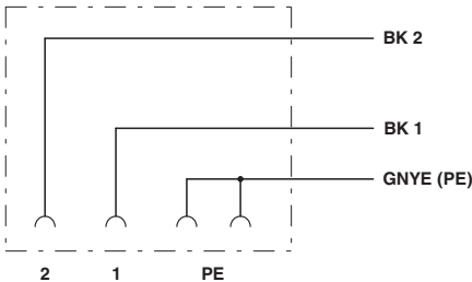
电路图
