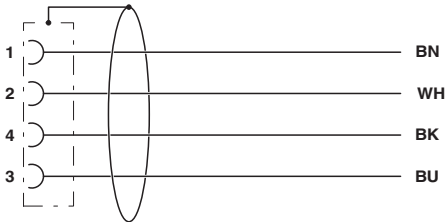
电路图
