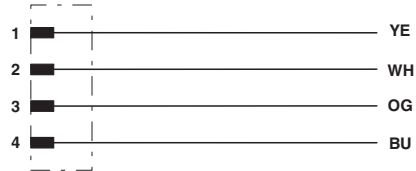
电路图
