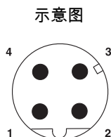
M12针式连接器引脚分配，4芯，D编码，插头侧
