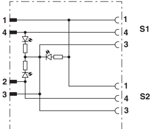
电路图
