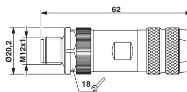
尺寸图
