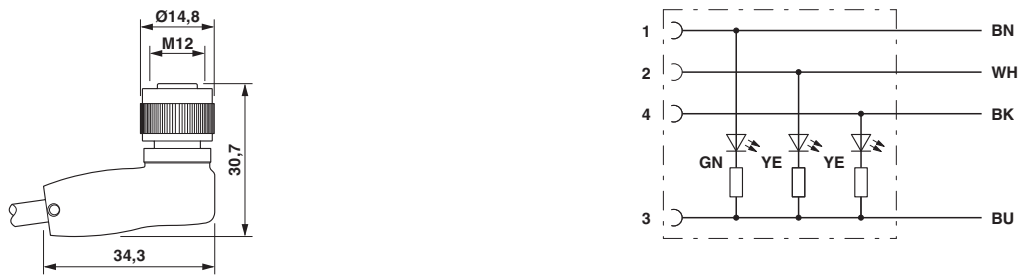
M12针式和M12孔式的触点分配
