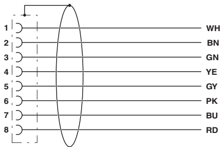
电路图
