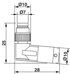
尺寸图
