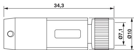
尺寸图
