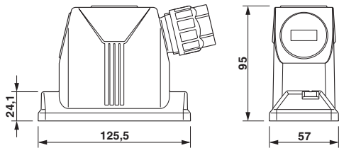
尺寸图
