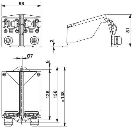
尺寸图
