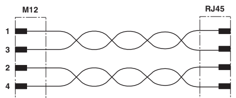
电路图
