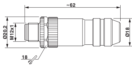
尺寸图
