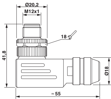
尺寸图
