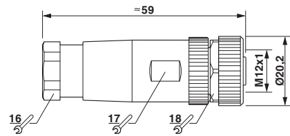
尺寸图
