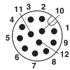
M12插头引脚分配，12芯，A编码，插头侧视图
