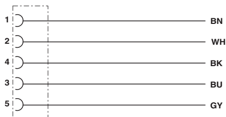
电路图
