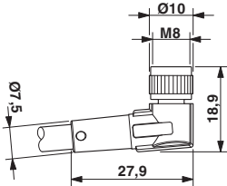
尺寸图
