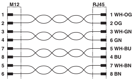
电路图
