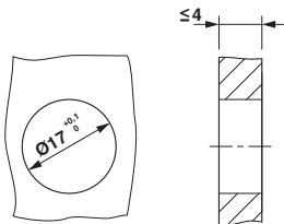
尺寸图
