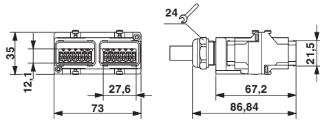
尺寸图
