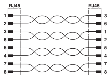
电路图
