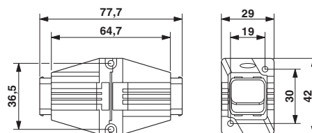
尺寸图
