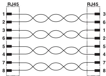
电路图
