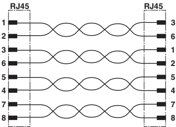
电路图
