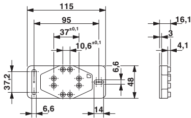
尺寸图
