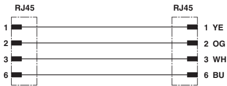
电路图
