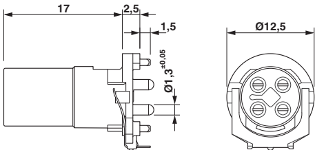
尺寸图
