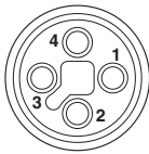
M12孔式引脚分配，4位，T编码，孔式连接器侧视图
