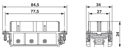
尺寸图
