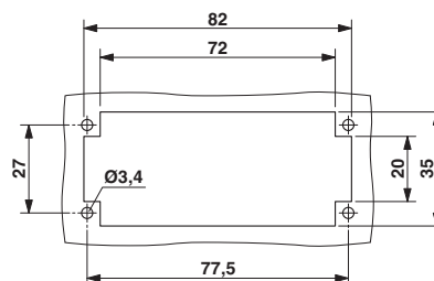
尺寸图
