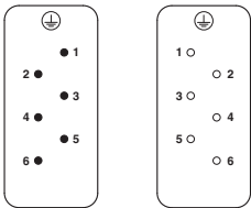
示意图
