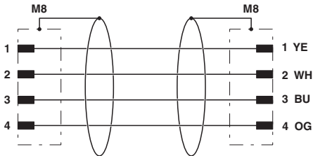
M8针式连接器触点分配
