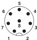
M12针式连接器引脚分配，8芯，A编码，插头侧视图
