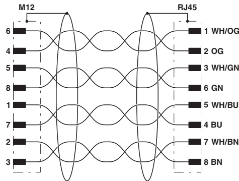
电路图
