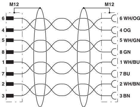
M12针式和M12孔式连接器的触点分配
