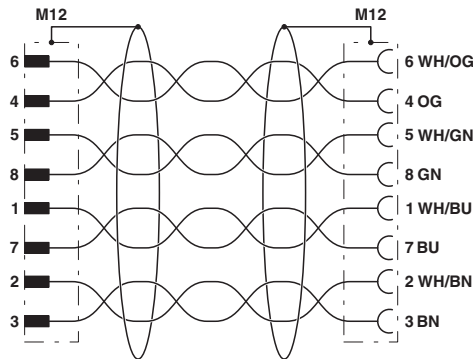
M12针式和M12孔式连接器的触点分配
