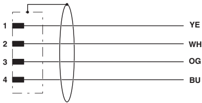
电路图
