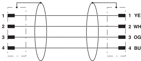
电路图
