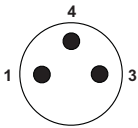
M8针式连接器引脚分配，3芯，插头侧视图
