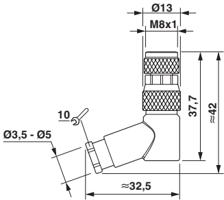
尺寸图
