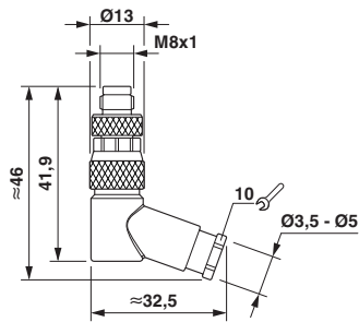
尺寸图
