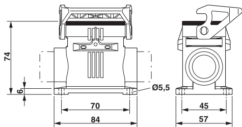
尺寸图
