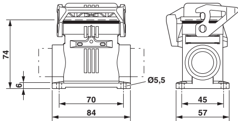
尺寸图
