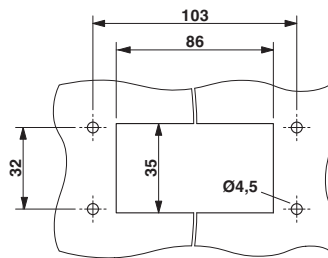
尺寸图
