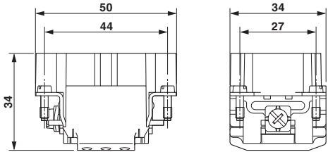
尺寸图
