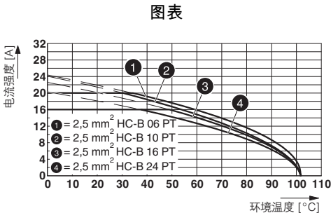
2.5 mm 2 电缆的衰减曲线图
