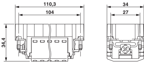
尺寸图
